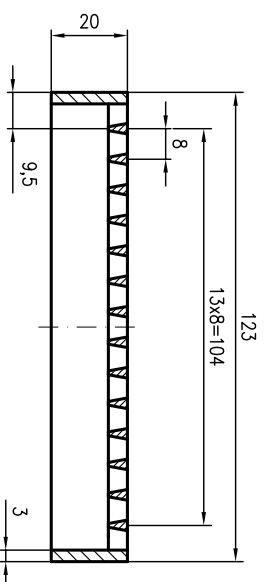
Schnitt A-A (123er Rost)
