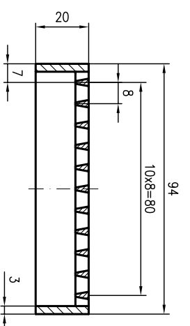
Schnitt A-A (94er Rost)
