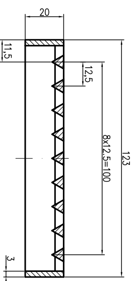
Schnitt A-A (123er Rost)
