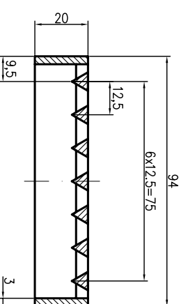
Schnitt A-A (94er Rost)
