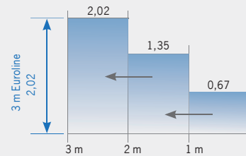
3 m-Strang Euroline leitet 2,02 l/s ab (siehe Tabelle)
